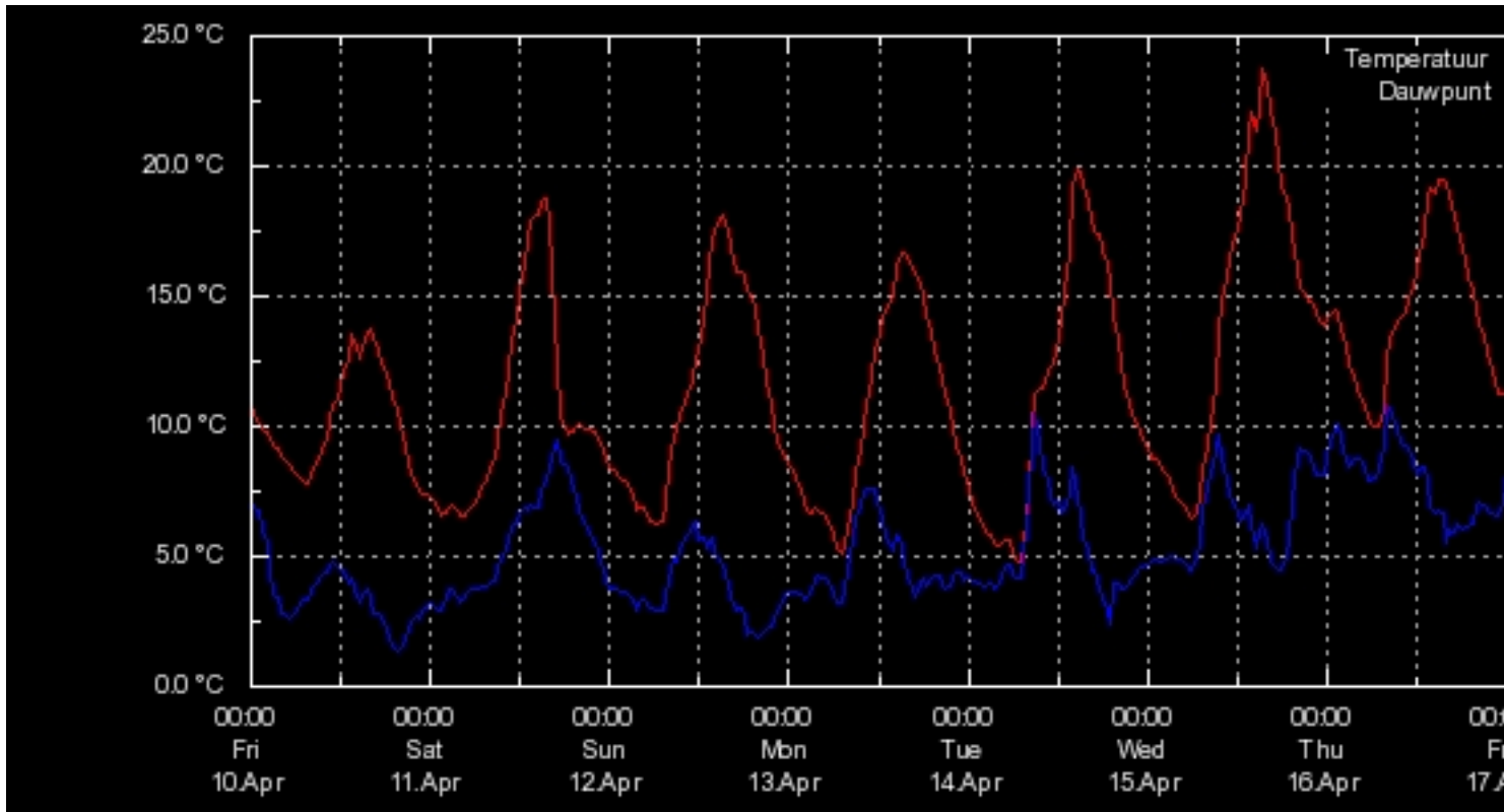
Buitentemperatuur - dagelijkse minima en maxima van de afgelopen 4 weken
